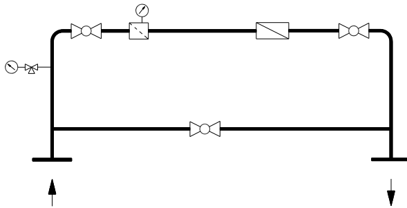
9. ábra Mérő állomás
