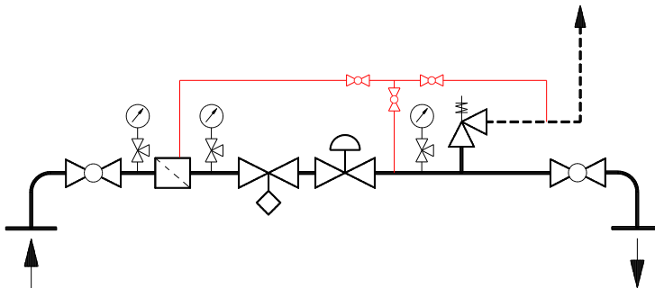
1. ábra Egy szabályozóág kialakítás
