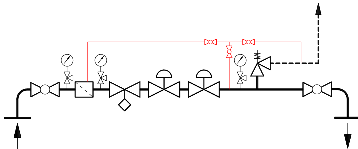
2. ábra Egy szabályozóágas, soros kapcsolású kialakítás
