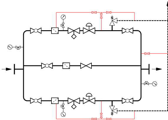
3. ábra Két szabályozóágas, párhuzamos kapcsolású kialakítás
