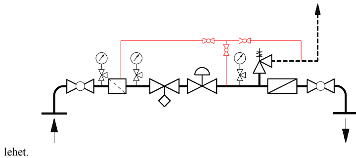
5. ábra Egy szabályozóágas, gázmérős kialakítás
